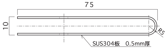
平面図
