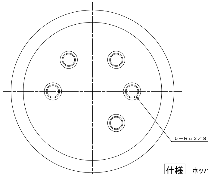
蓋加工図
