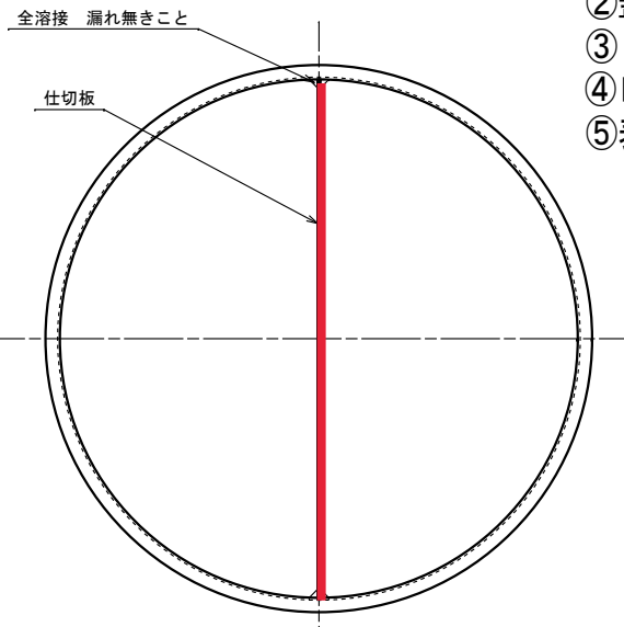
タンク上部 (平面図)
